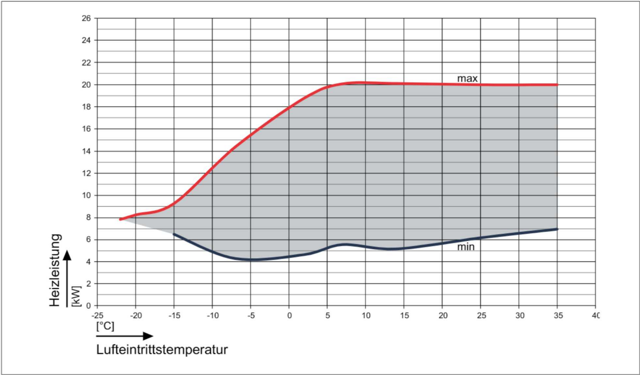
Abb. 8: Heizleistung CHA-16/20 bei einem Vorlauf von 65 °C
